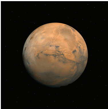
Mars
