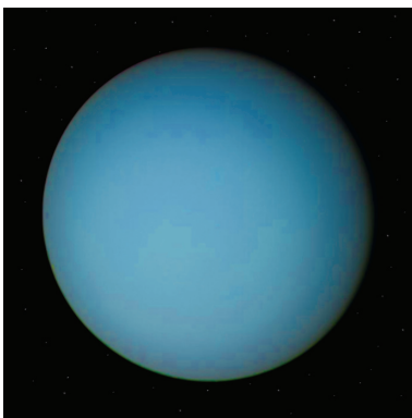
Uranus
