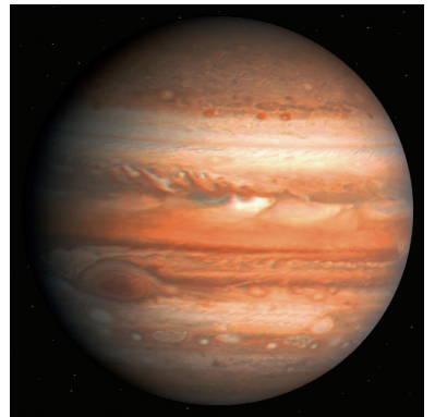
Jupiter
