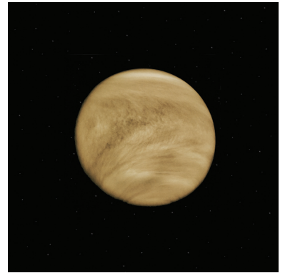
Venus
