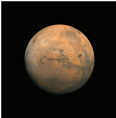
Mars
