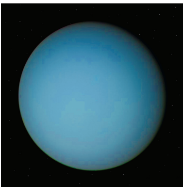
Uranus
